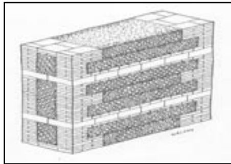
Opus mixtum
