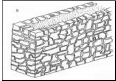
Opus incertum
